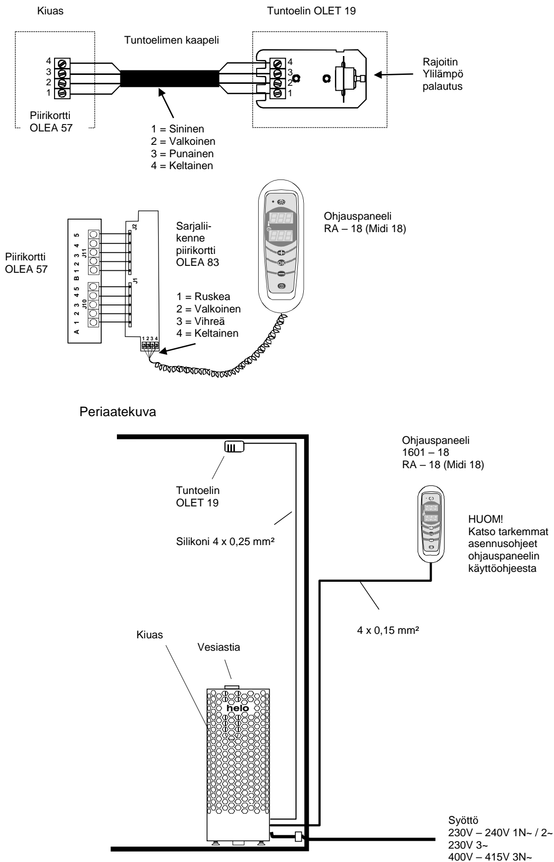
Kuva 6 Periaatekuva kytkennästä
