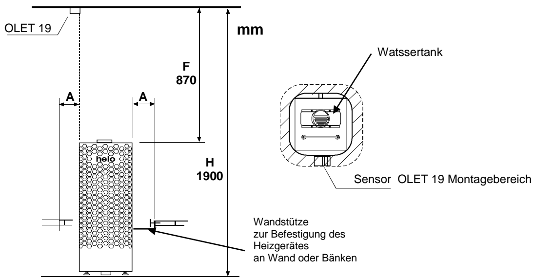
Abbildung 2 Sicherheitsabstände
