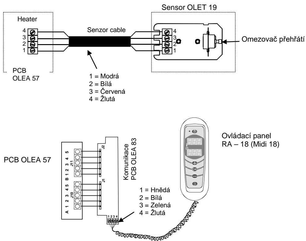
Schéma zapojení
